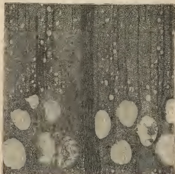
Fig. 5. - Roble ( Quercus Sessiflora , Smith). - Sección transversal. Aumento 30 diámetros.
